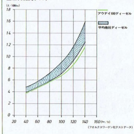
■燃料消費テスト
