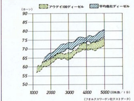
■室内騒音測定テスト
