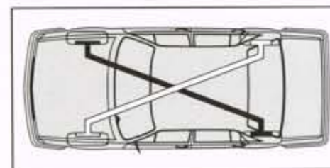
Beim Diagonal-Zweikreis-Bremssystem bleibt auch bei Ausfall eines Bremskreises die Bremskraftverteilung zwischen Vorder- und Hinterachse unverändert. An beiden Achsen verbleibt eine Bremswirkung von 50%.
